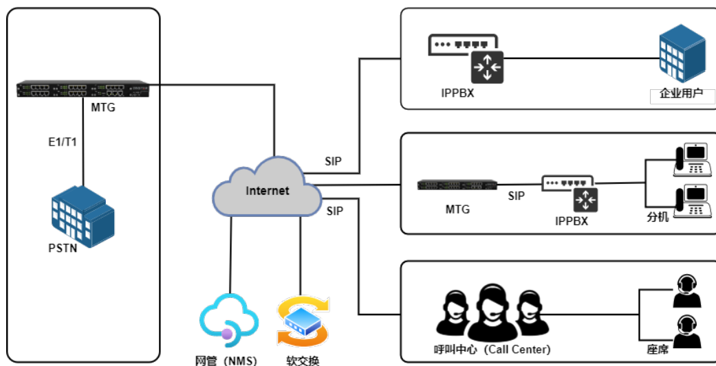
图 1-1-1 网络应用拓扑
